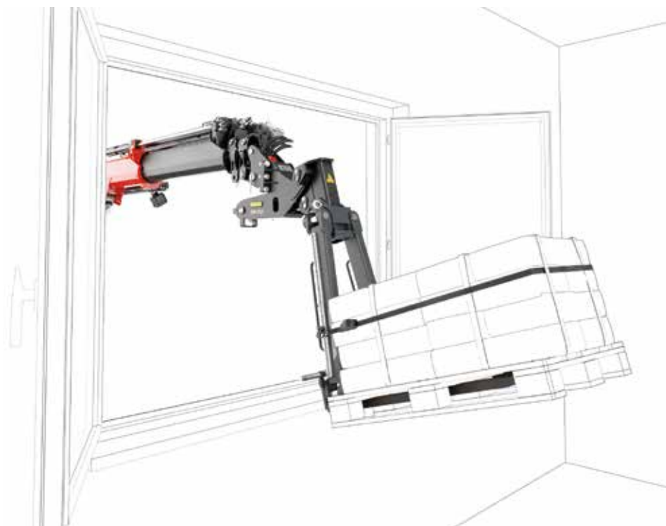
Kippbare Krangabel.
