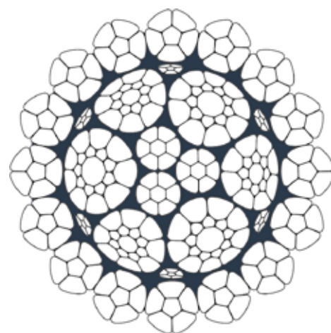
Graphik des Lazerlift-Seilquerschnitts.
